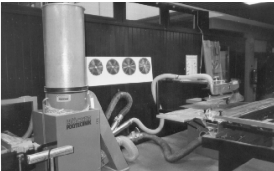
Bild 2: Entstauber zum Absaugen von stationären Holzbearbeitungsmaschinen in der Schule (Foto: Ludger Hohenberger)
